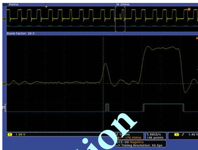
MagniVu 高解析度記錄提供 60 ps 的時序解析度，讓您能夠在數位波形上進行重要的時序量測。
