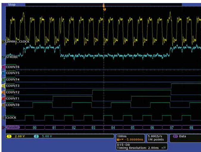
MSO 系列提供 16 個整合的數位通道，可讓您檢視與分析和時間相關的類比和數位訊號。
