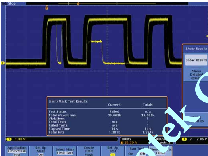
「極限測試」會顯示使用標準波形建立並對照訊號進行比較的遮罩。顯示結果表示測試的相關統計資訊。
