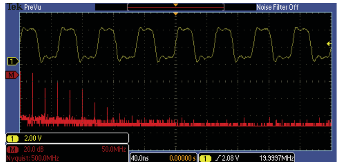
分析 – 脈衝訊號的 FFT 分析。一套全方位的整合分析工具可加速您設計效能的驗證。
