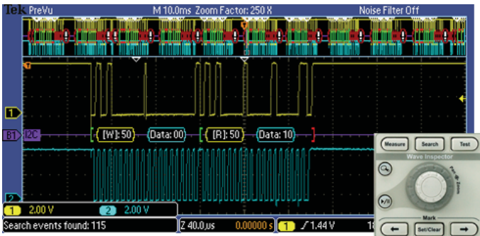
搜尋 – I 2 C 解碼顯示 Wave Inspector 搜尋位址數值 50 的結果，Wave Inspector 控制提供在檢視和瀏覽波形資料時前所未有的效能。
