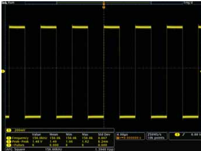
自動量測讀數提供的波形特性的可重複統計視圖。
